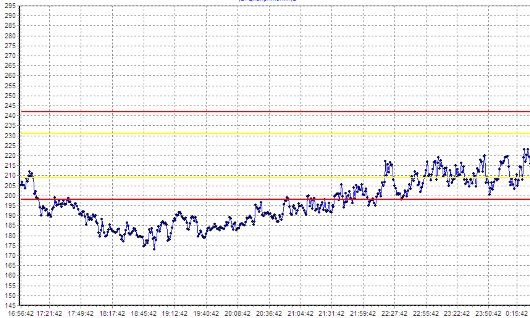
График діючої напруги ,Вцнапряження,В
